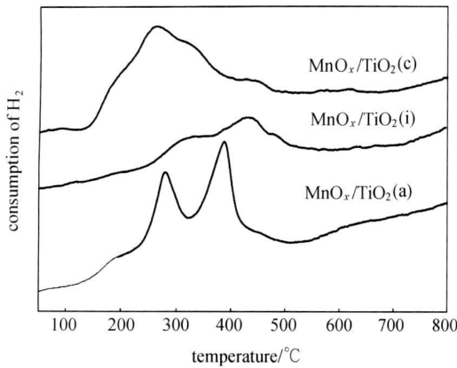
图 6 催化剂的 TPR 谱图
