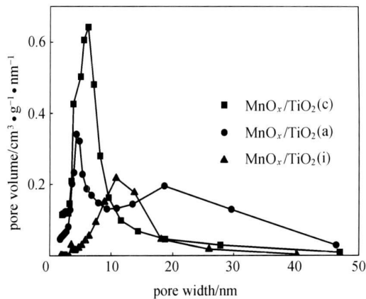
图 2 样品孔径分布
