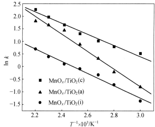
图 8 催化剂 Arrhenius 曲线
