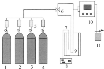
图 1 实验装置流程
