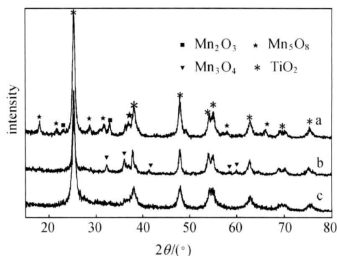
图4 催化剂的 XRD 图
