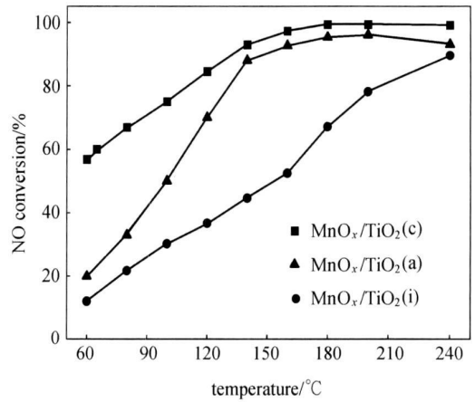
图 7 3 种方法制备的催化剂脱硝活性
