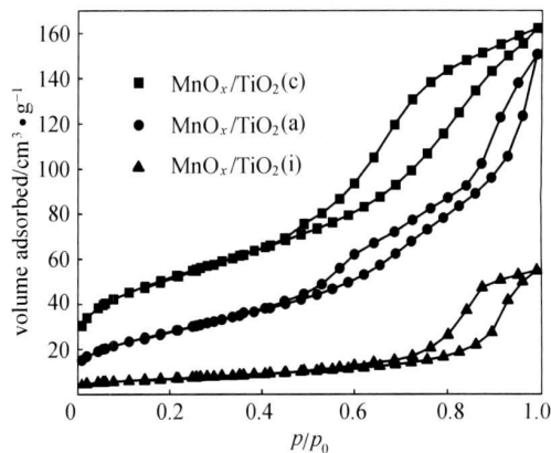
图 3 样品吸附-脱附等温线
