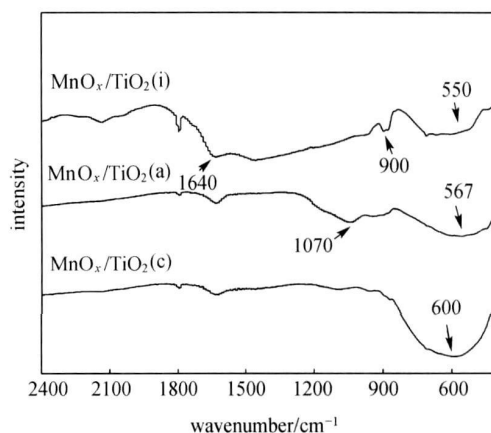
图5 样品 FTIR 谱图
